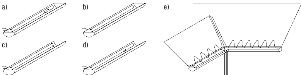
EXAMPLES OF LAYING ADPSV CABLE / PŘÍKLAD ULOŽENÍ KABELU ADPSV
