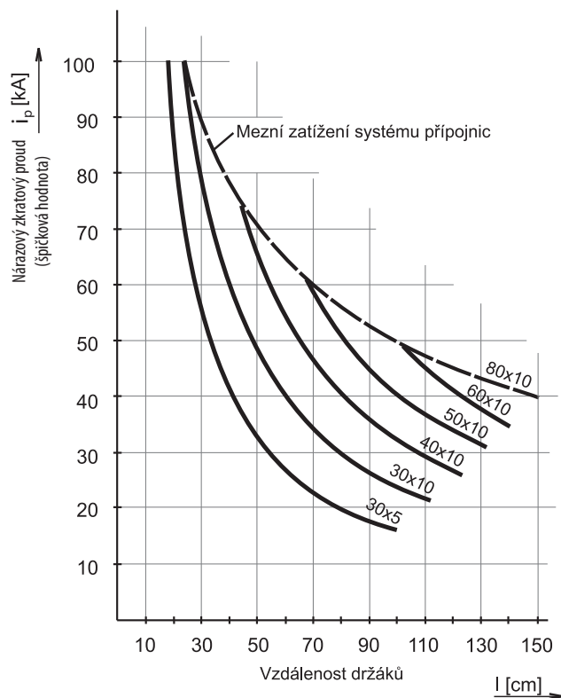
Systém přípojnic 100 mm
