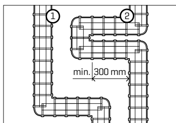
provedení záchytných ohybů na svislé trase
