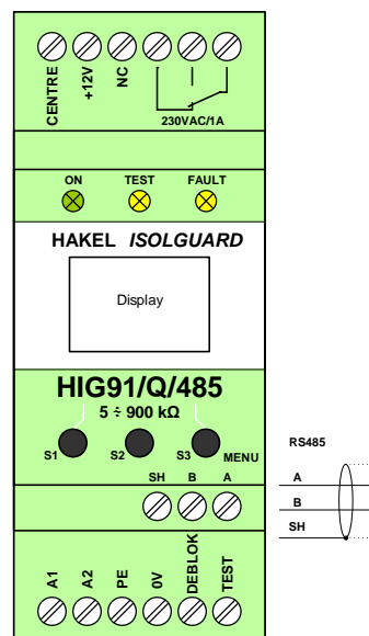
Zapojení svorkovnic
