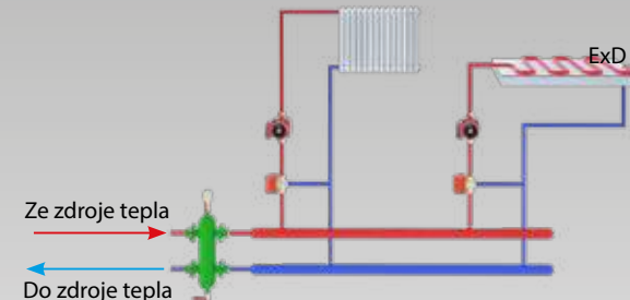
Schéma zapojení 4
