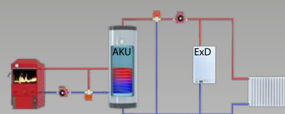
Schéma zapojení 2
