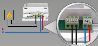
Ovládání kotle
