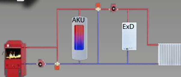
Schéma zapojení 2
