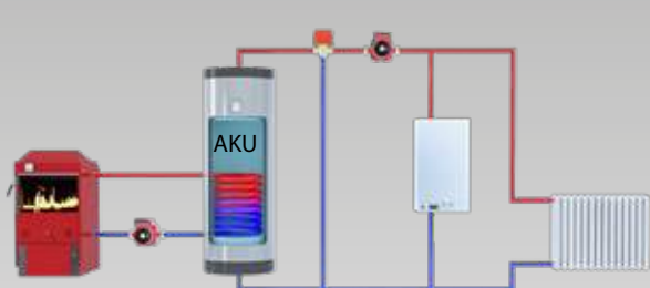
Schéma zapojení 3
